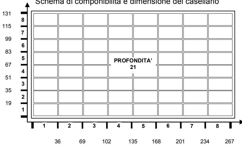
Schema di componibilità e dimensione del casellario
